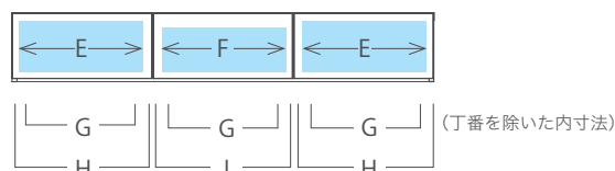
正面図
