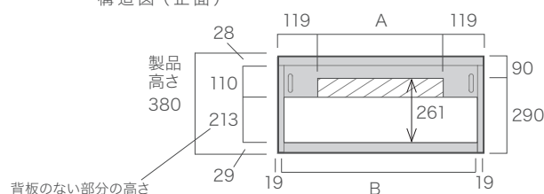
構造図 (正面)
