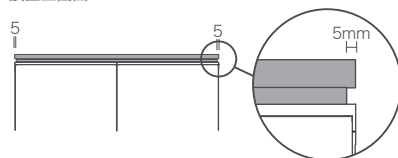
設置正面図
