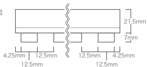
上面図
