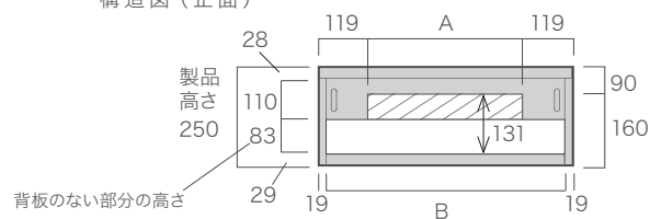
構造図 (正面)
