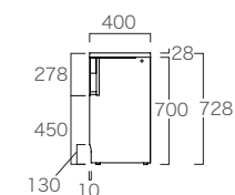
右設置用 側面図
