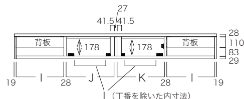
正面図(構造図)
