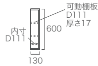
側面図
