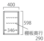
正面図
